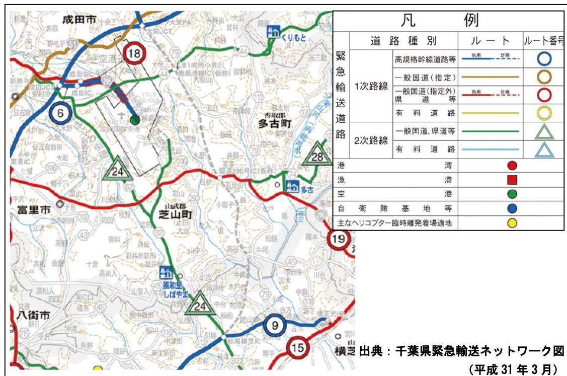
図 2-4 芝山町における緊急輸送道路
