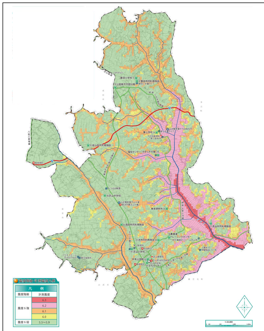
図2-2 揺れやすさマップ
