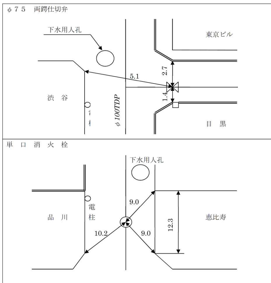
図－２ オフセット図
